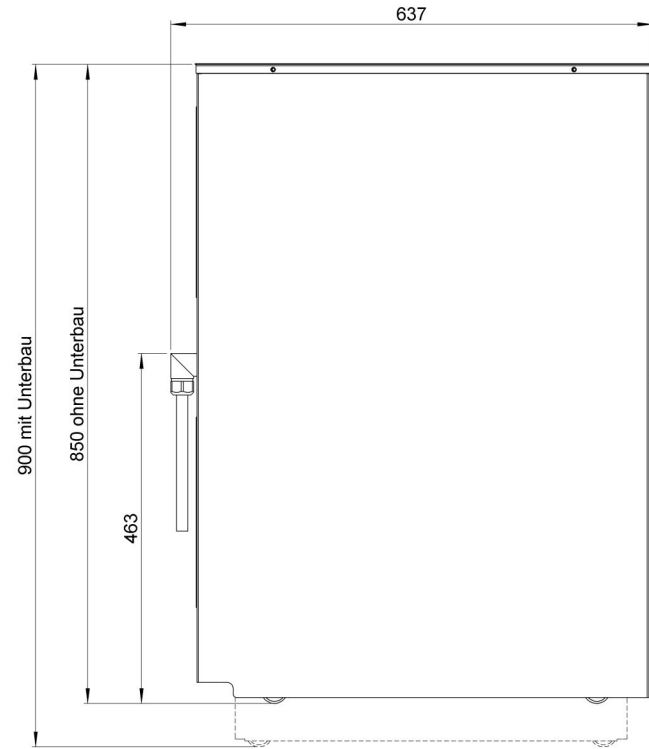
Korbhebeautomatik ausgefahren Masstab 1:10
